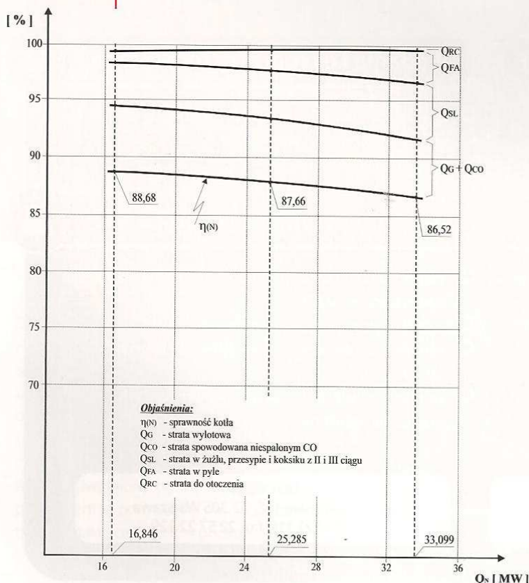
Rys. 1. Charakterystyka energetyczna kotła typu WR25-014SC Nr 4 Źródło: Sprawozdanie z pomiarów energetycznych kotła typu WR25-014SN nr 4 zainstalowanego w Miejskim Przedsiębiorstwie Energetyki Ciepłej we Włocławku, s.11.
